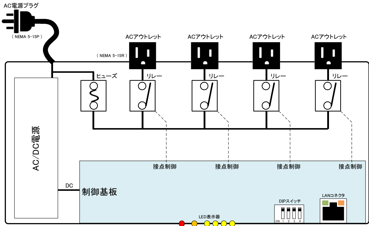
Fig.5 内部構成図
