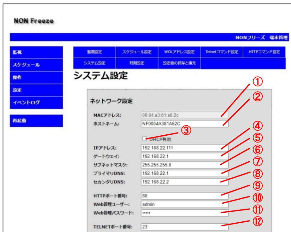
Fig.29 システム設定画面（ネットワーク設定）
