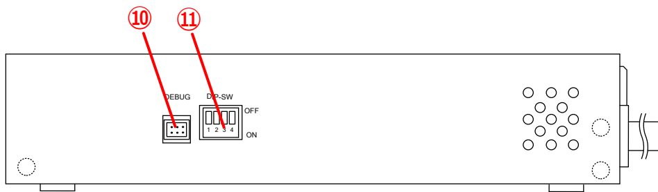
Fig.4 左側面図
