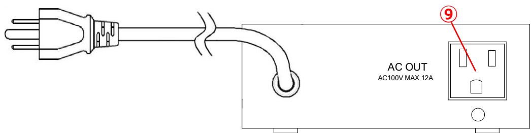
Fig. 18 電源出力対応図（背面）
