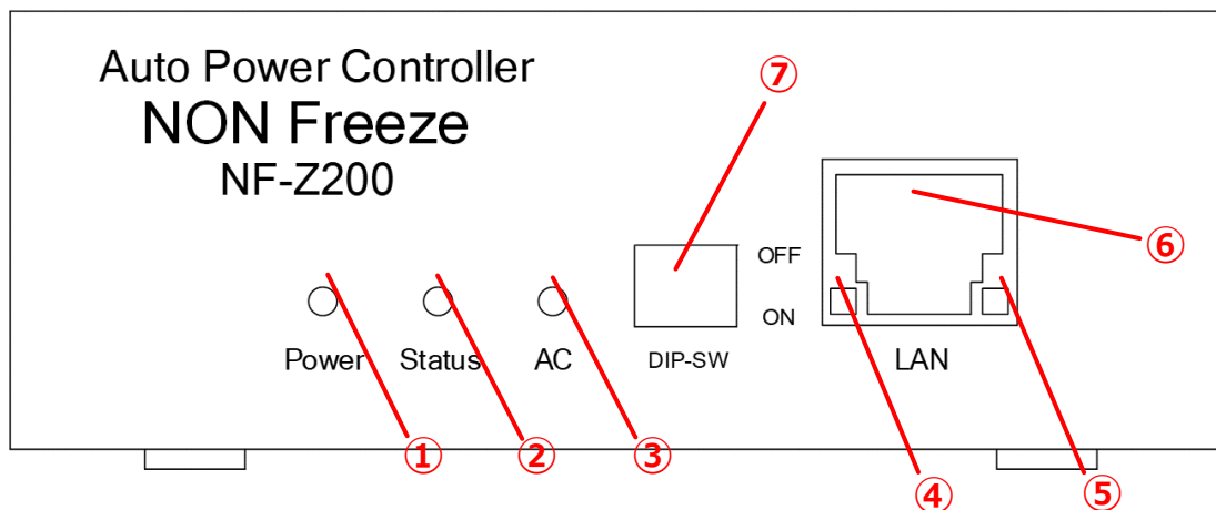
Fig. 2 前面図
