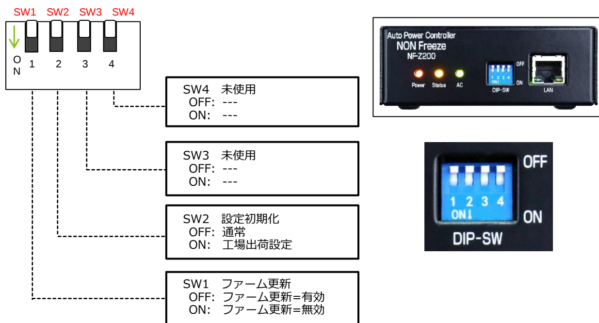
Fig. 8 DIP スイッチ設定
