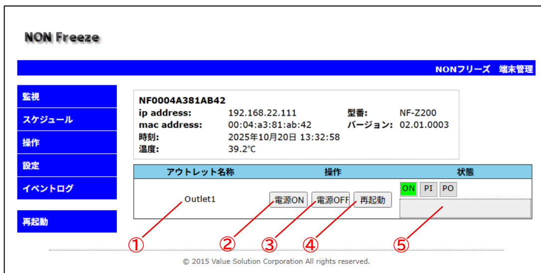
Fig. 21 操作画面
