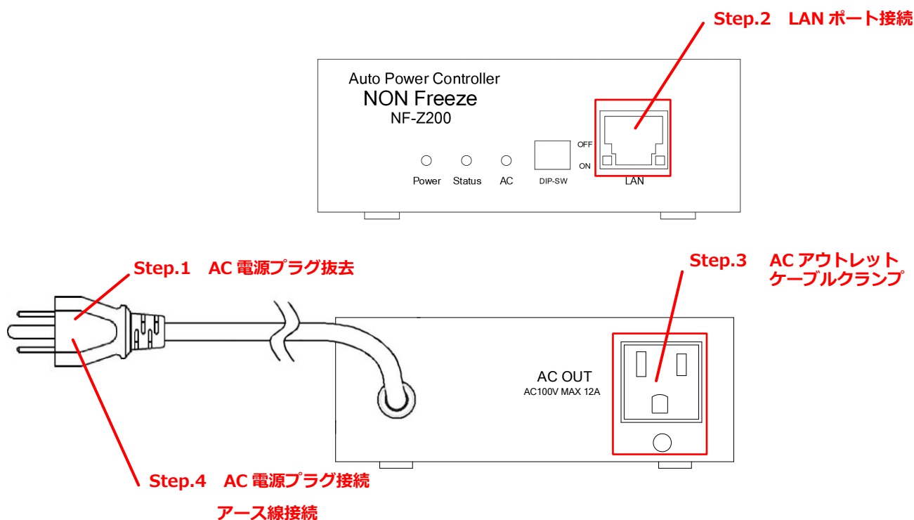
Fig. 7 接続説明図
