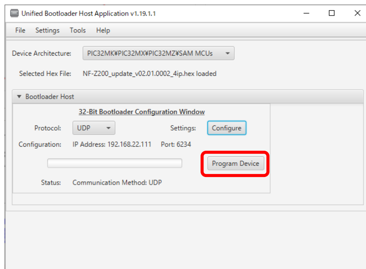
Fig. 49 更新実行
