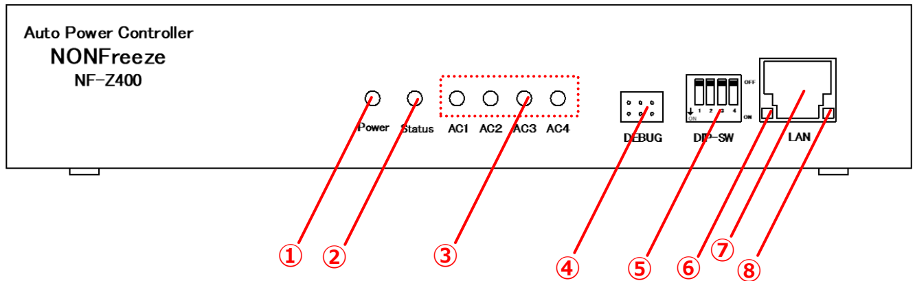
Fig. 2 前面図
