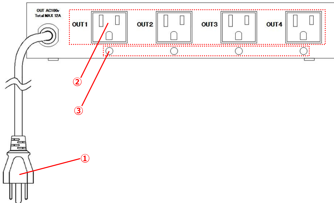
Fig. 3 背面図
