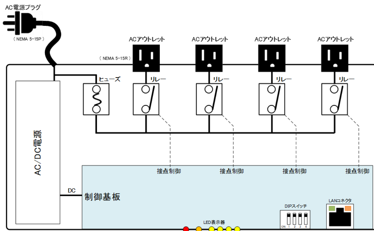
Fig. 5 内部構成図
