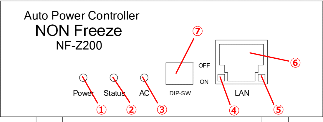
Fig. 2 前面図
