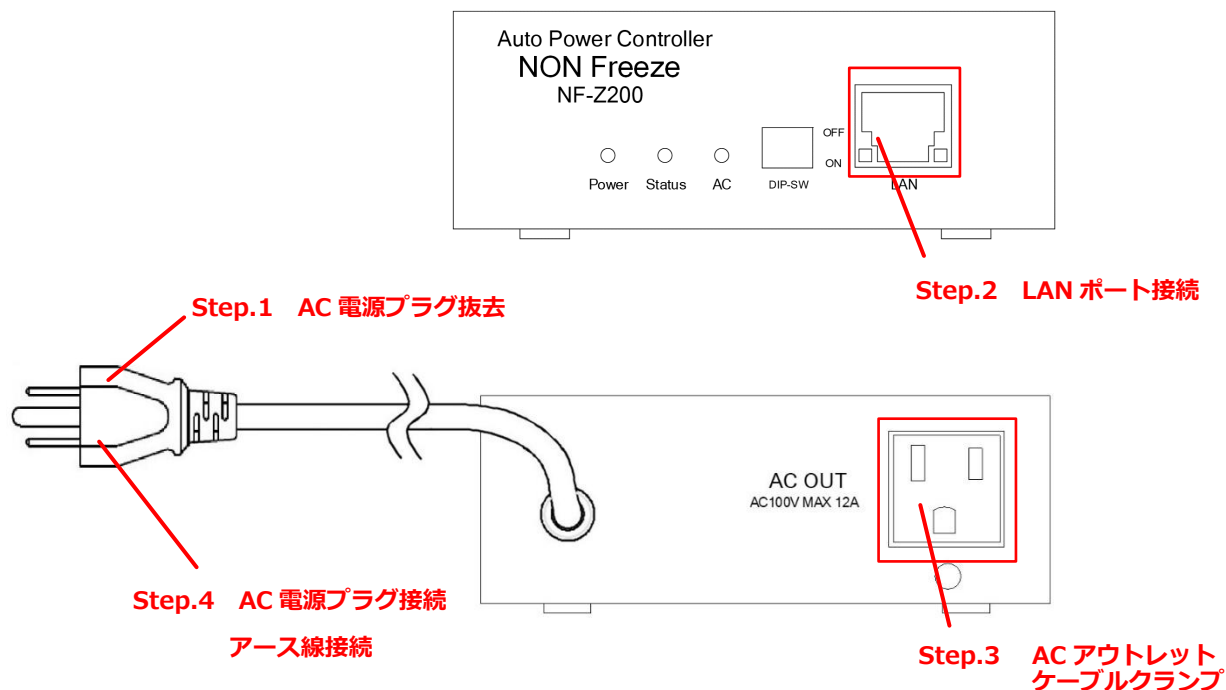
Fig. 7 接続説明図
