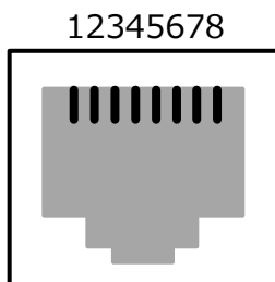
Fig. 40 LAN ポートピン配列
