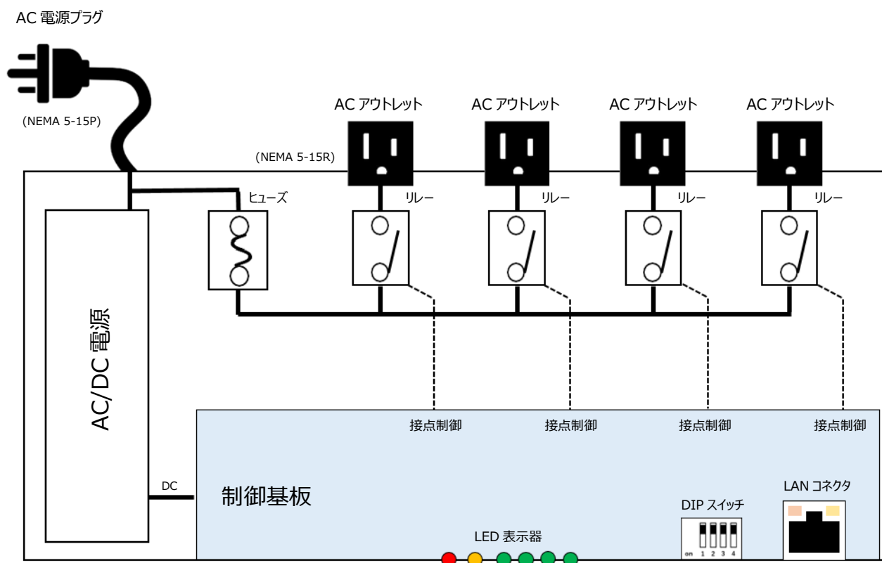
Fig. 5 内部構成図
